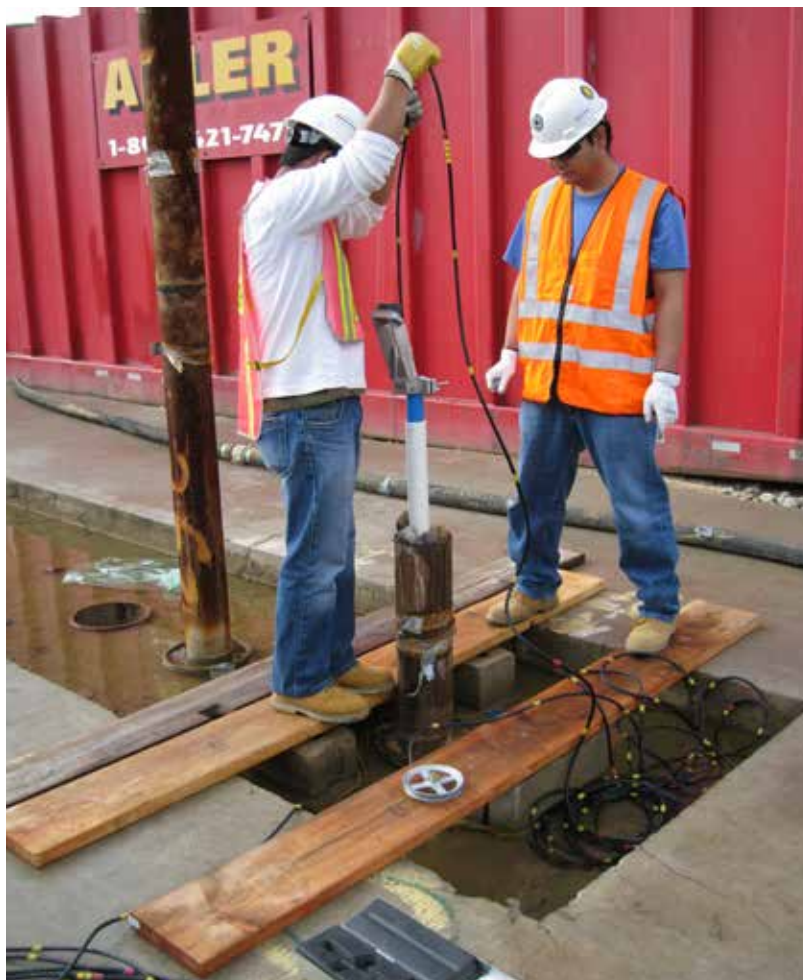
Fig. 13. Ispezione visiva con telecamera all'interno dei carotaggi
