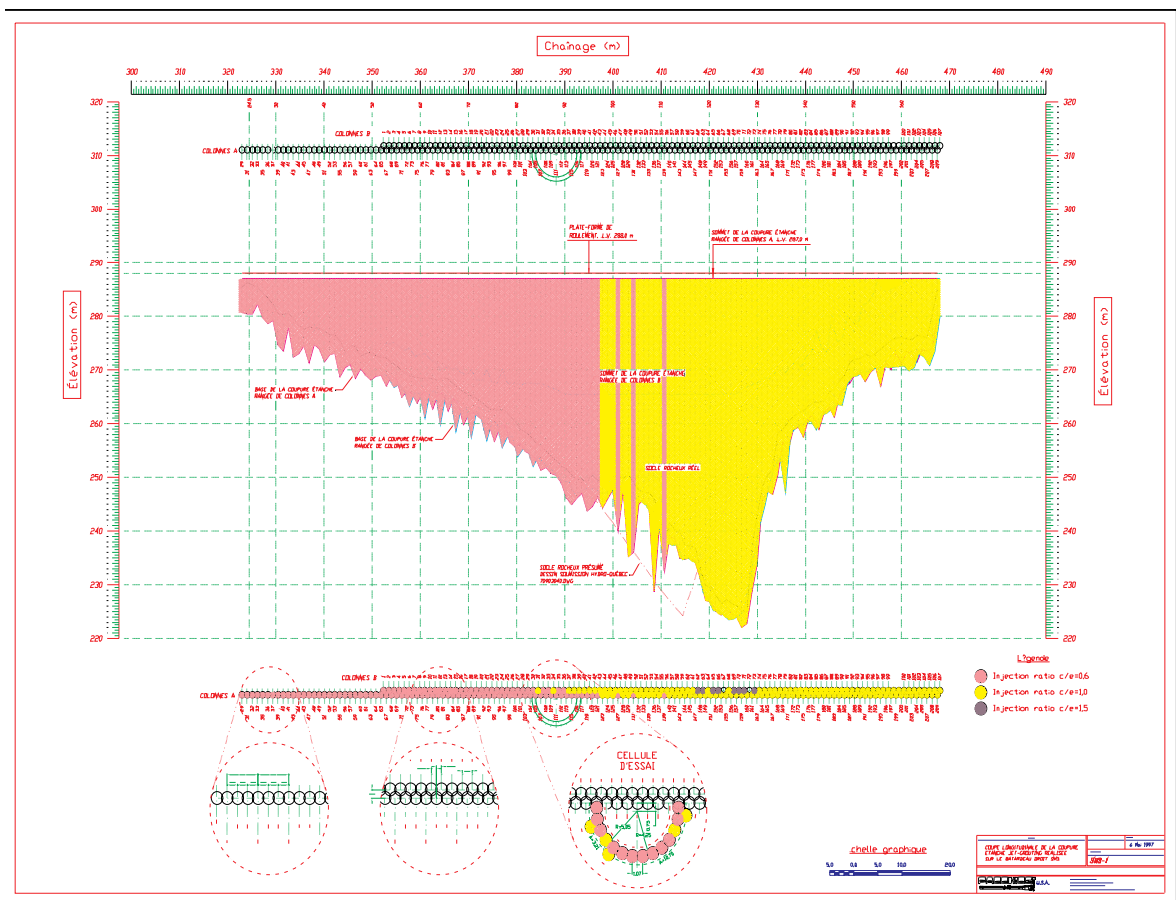
Fig. 4. Grafico rappresentante le caratteristiche delle colonne Jet Grouting.
